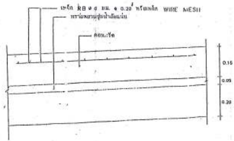
รายละเอียดถนนคอนกรีตผิวหน้า
