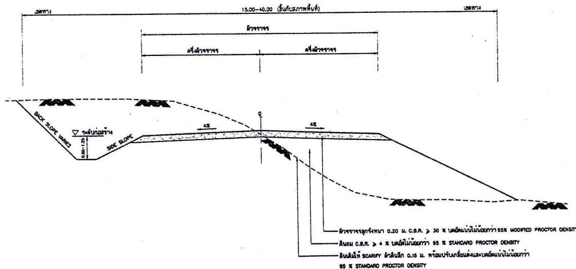
รูปตัดคั่นทางแบบดินตัดและดินถม มาตราส่วน 1 : 50
